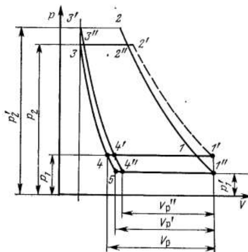
1 – rasm. Kompessor silindrida havoni so‘rish, siqish va haydash jarayonlarining indikator diagrammasi
