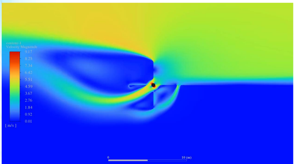
Рис. 4. Контур скорости V=6 м/с.
