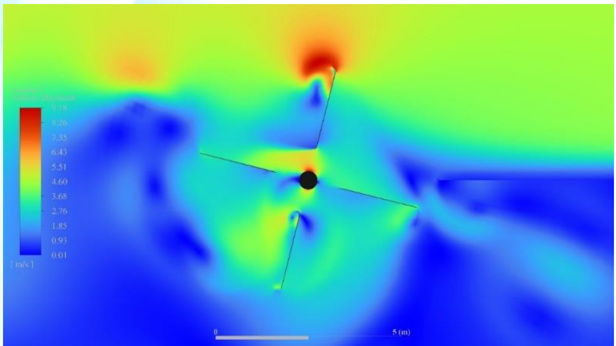
Рис. 3. Контур скорости V=5 м/с.
