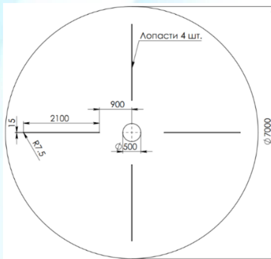
Рис. 1. Двухмерная геометрия ветряной турбины (вид сверху)
