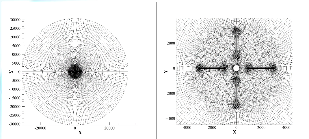
Рис. 2. Неструктурированная расчетная сетка конечных объемов.
