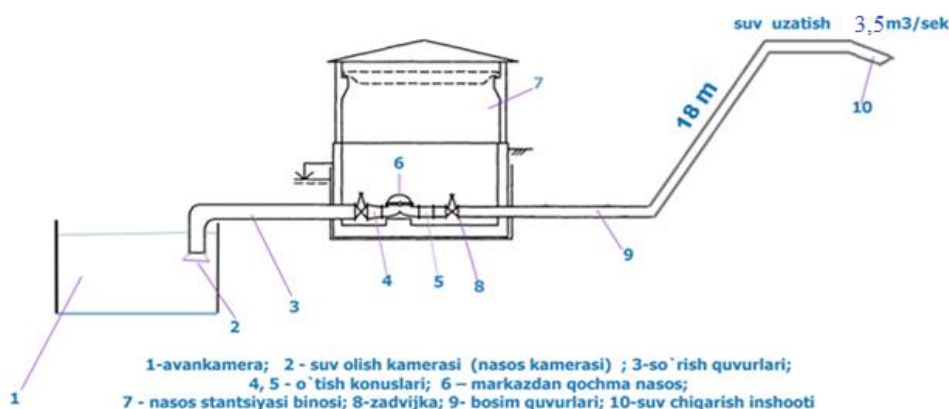
"Paykent" nasos stansiyasining texnologik jarayon sxemasi
