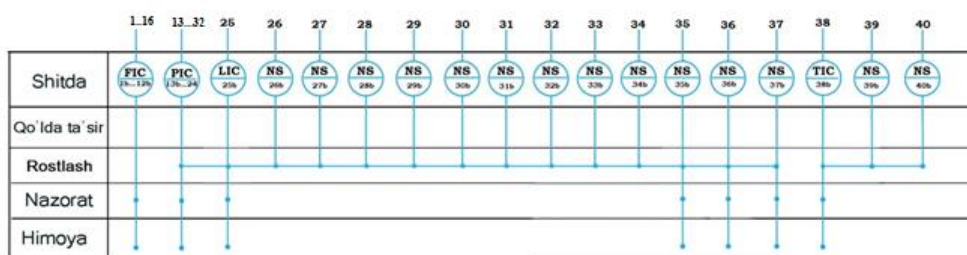
2-rasm Nasos stansiyasini avtomatlashtirish funksional sxemasi
